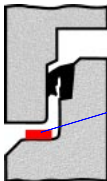
aufgelegtes EGOTAPE 243 vor der Schachtring-Montage
