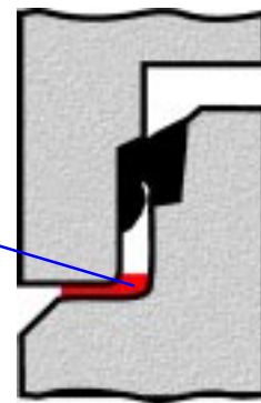
aufgesetzter oberer Schachtring mit verformtem lastübertragendem EGOTAPE 243
